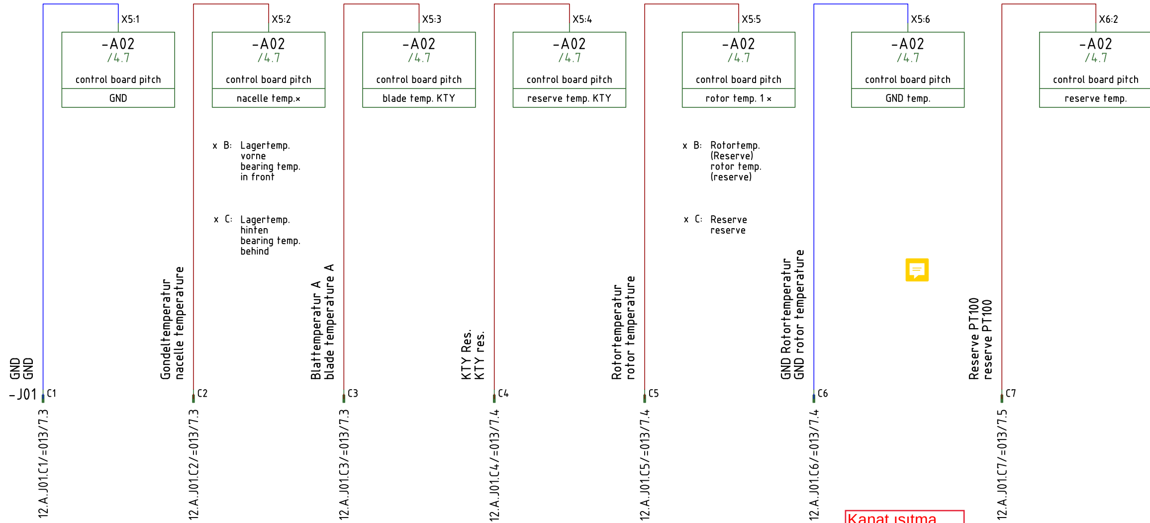
Rotorunterverteilung rotor subdistribution
